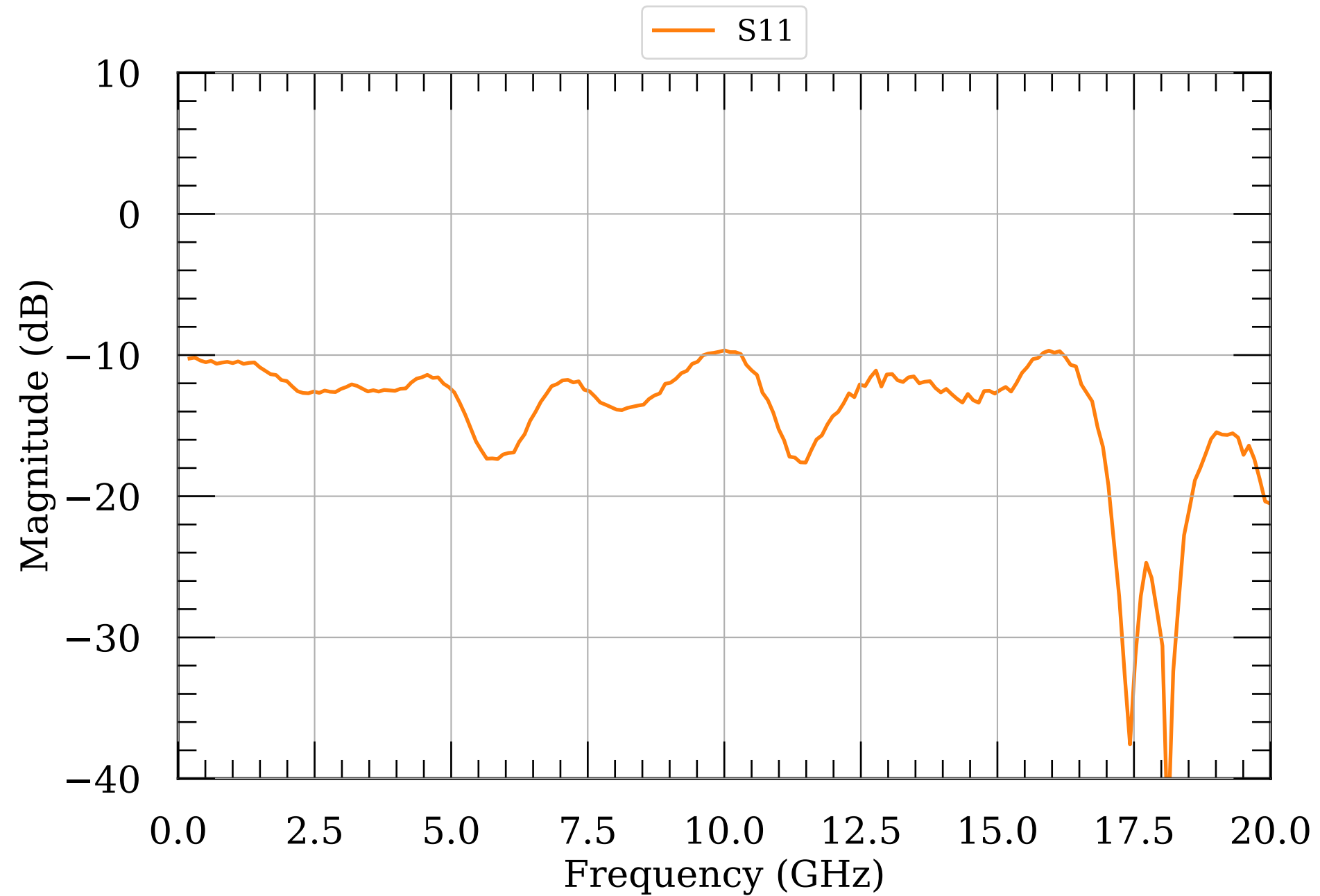
LNA S-params module025v2
